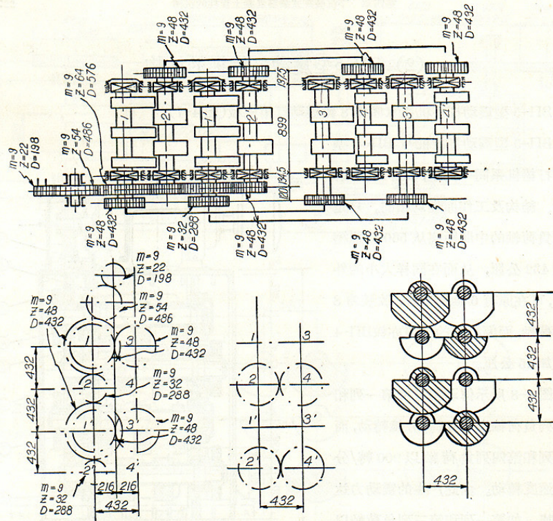
图 4-8 BII-5 型震动打樁机齿轮传动图
