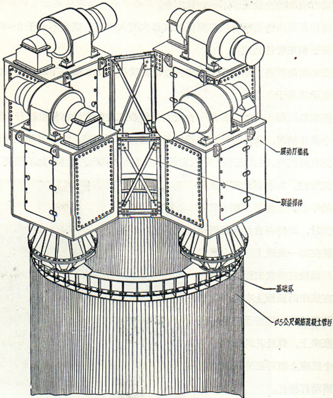
图 4-22B 四台同步工作震动打桩机示意图
