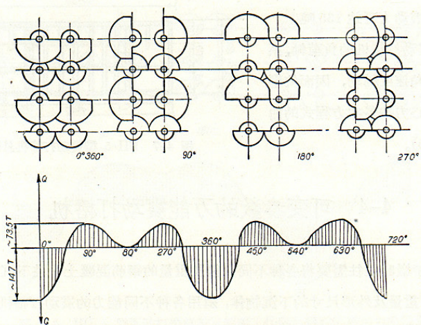
图 4-9 BII-5 型震动打樁机震动力变化曲线图
