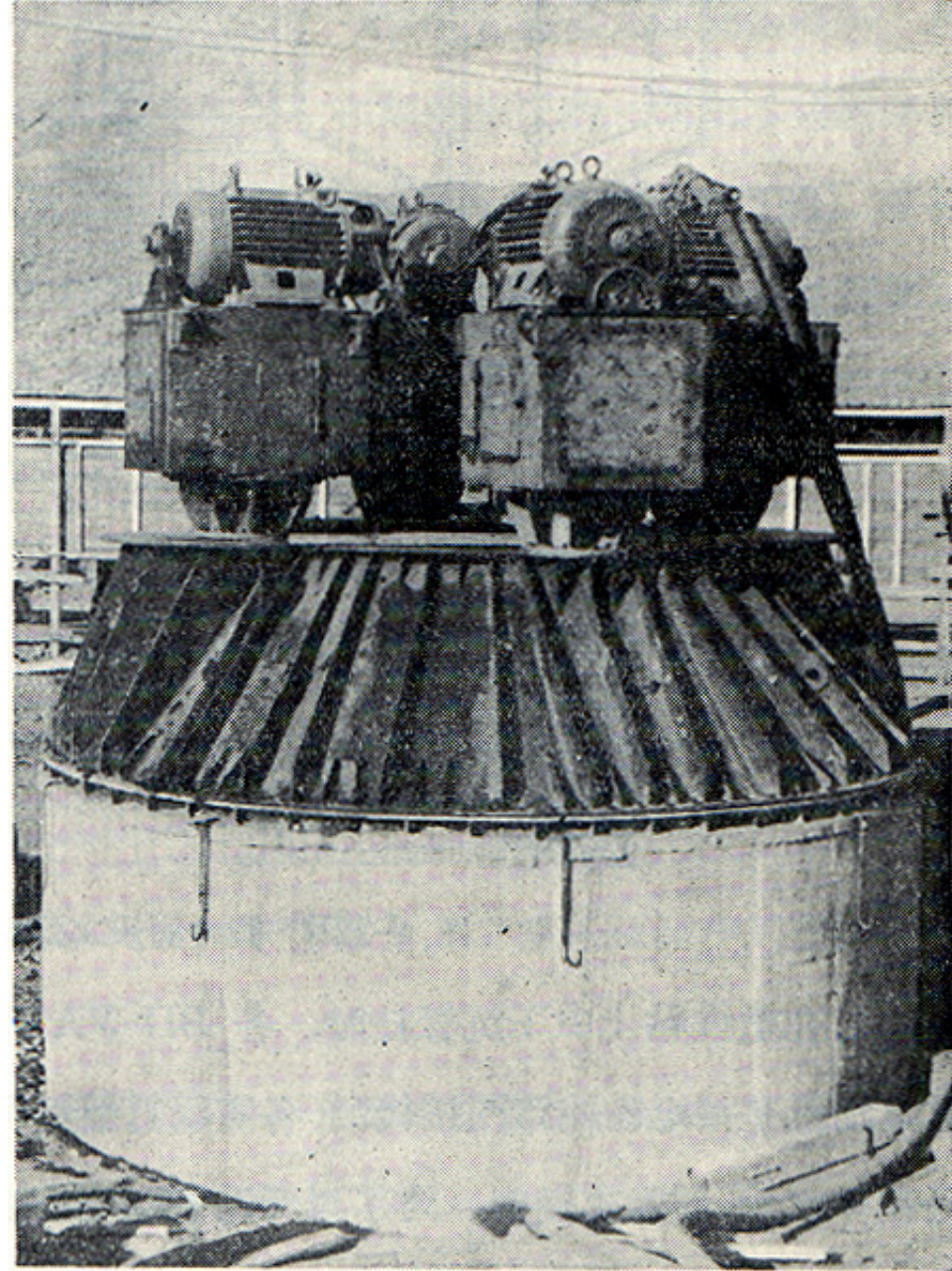
图 4-22A 四台同步工作震动打桩机正在下沉直径 5 公尺的管柱
